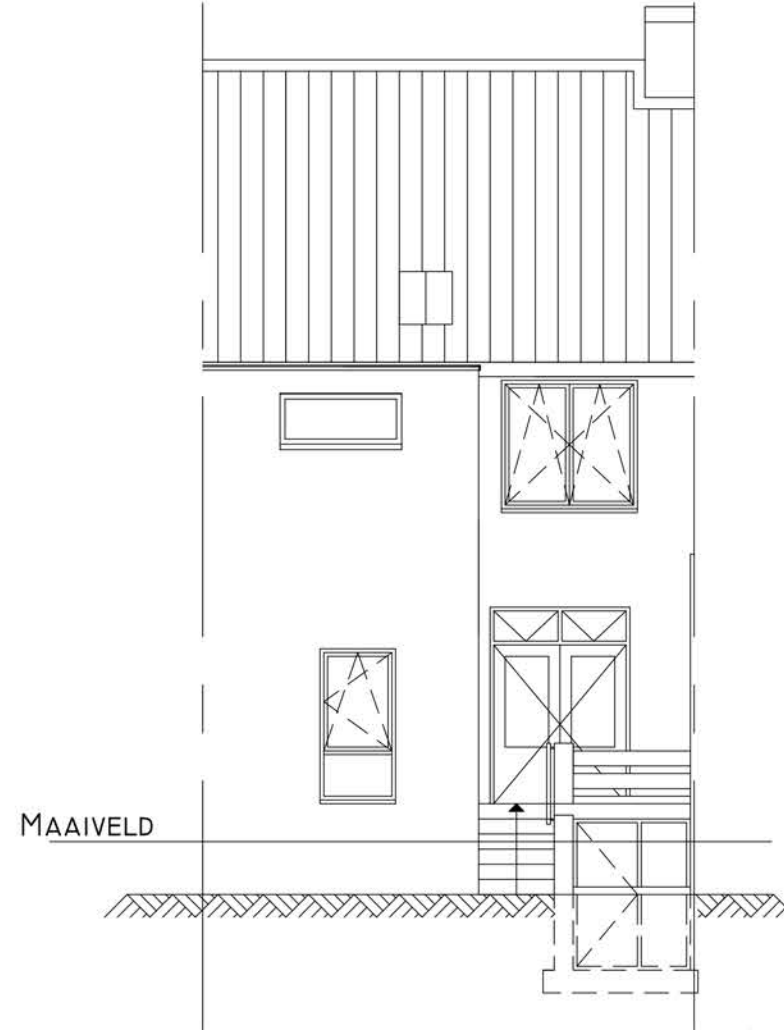
ACHTERAANZICHT
