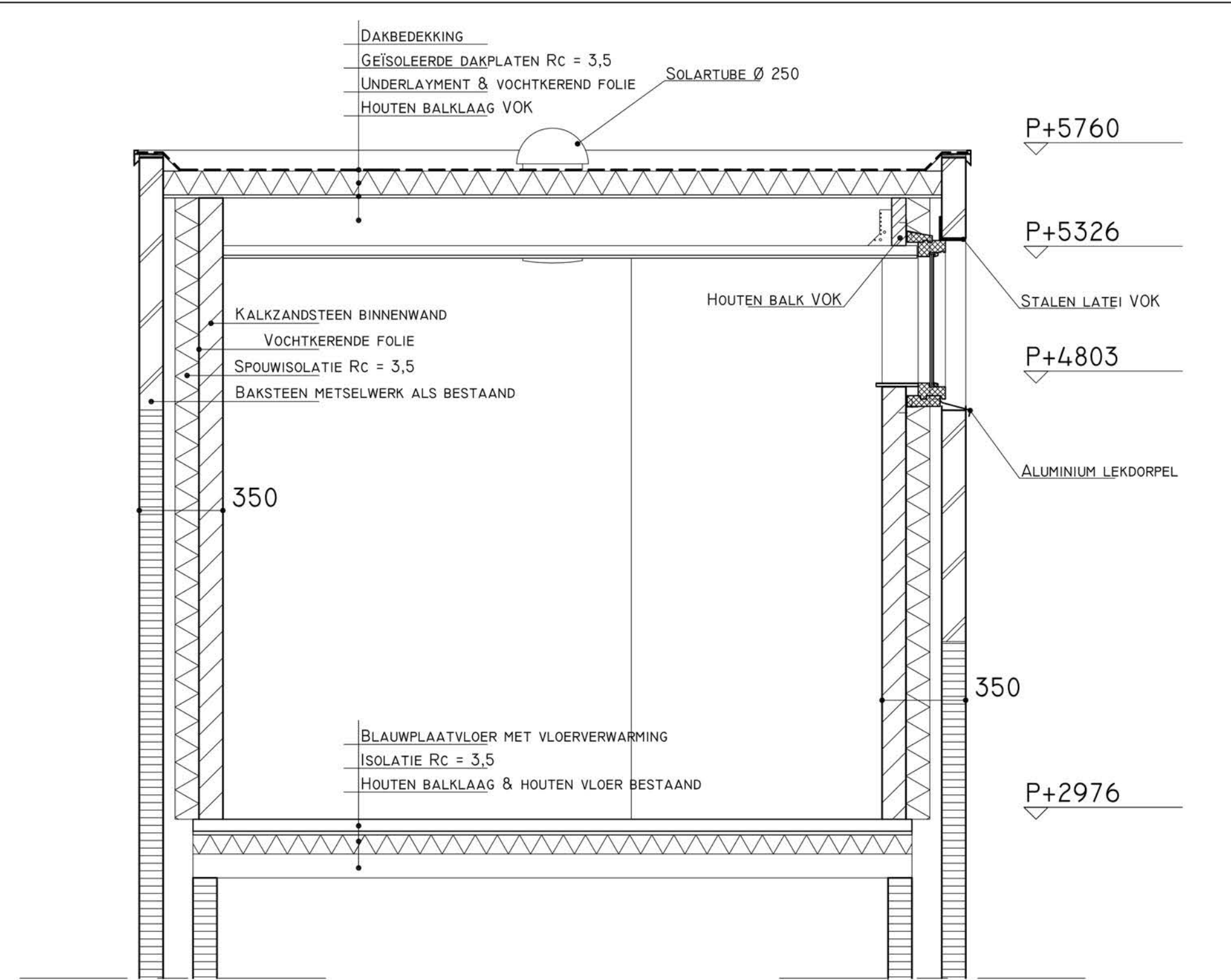
DOORSNEDE B-B' 1:20
