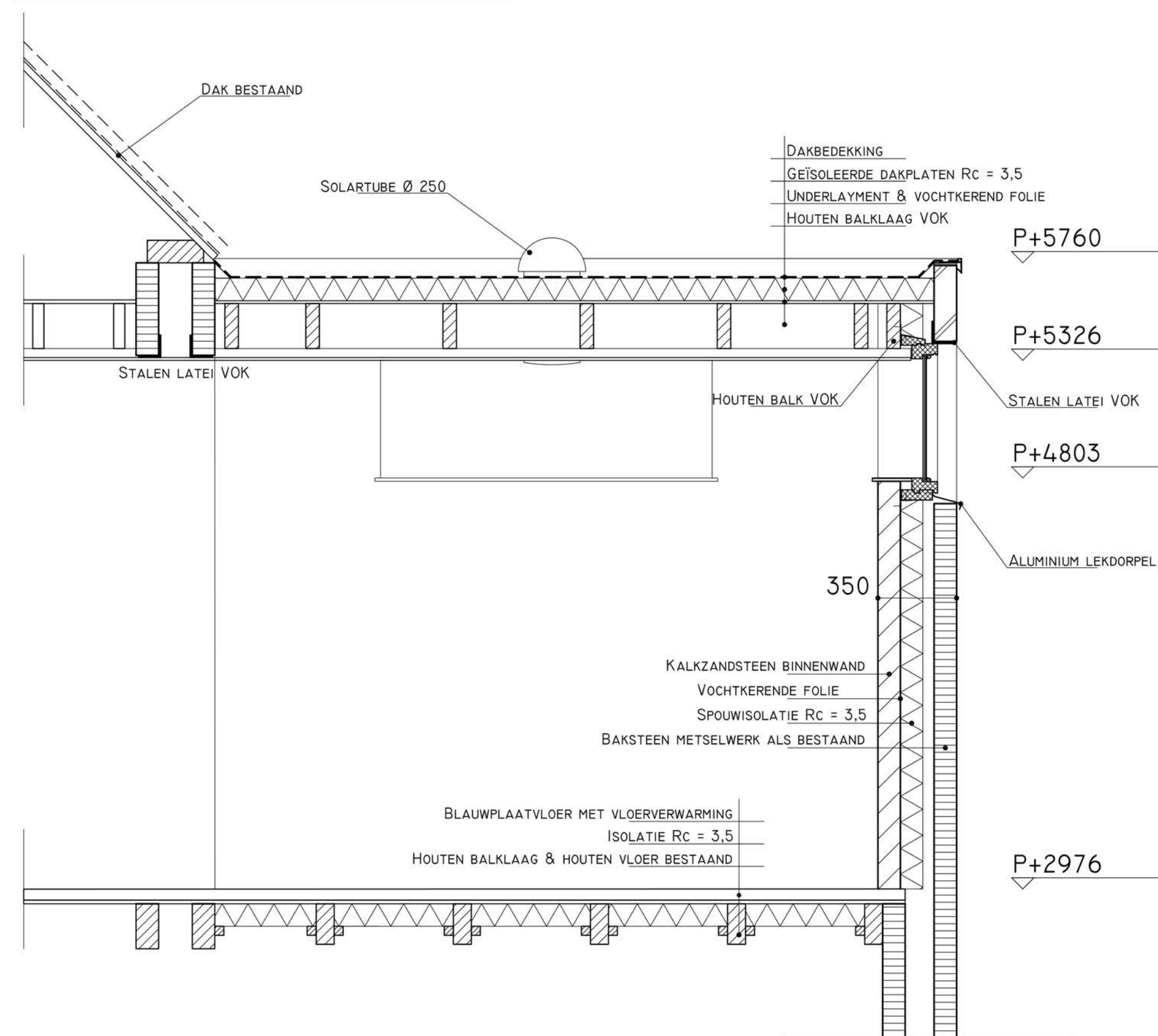
DOORSNEDE C-C' 1:20
