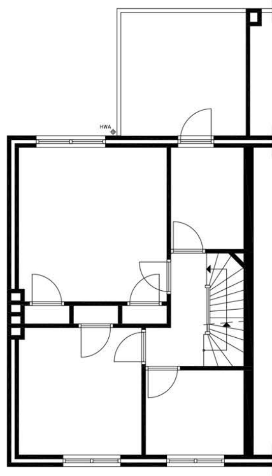
1E VERDIEPINGSVLOER BESTAAND
