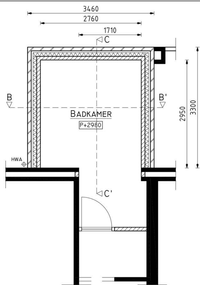
BADKAMER NIEUW 1:50
