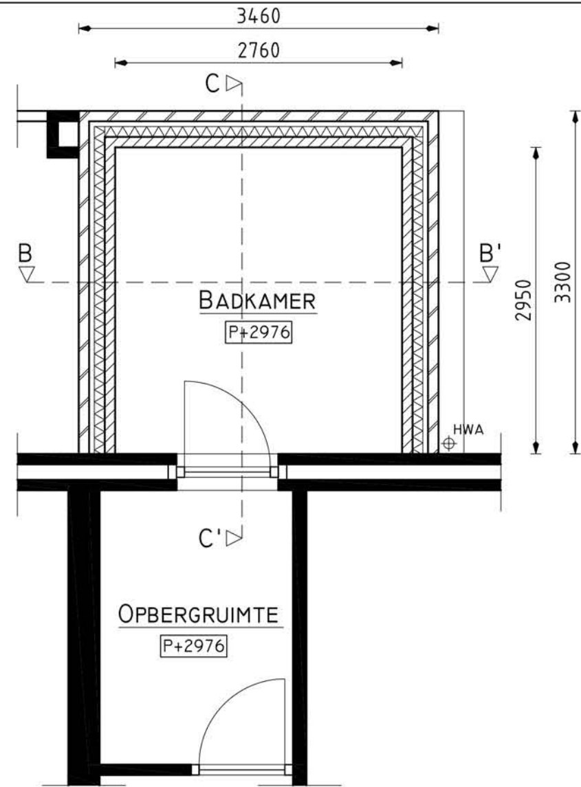
BADKAMER NIEUW 1:50
