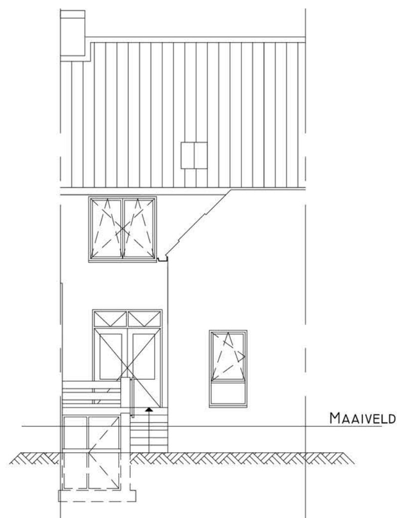
ACHTERAANZICHT
