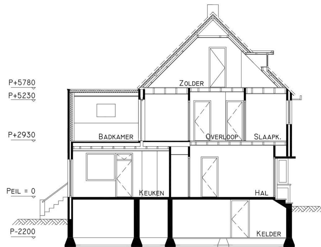
DOORSNEDE A-A'
