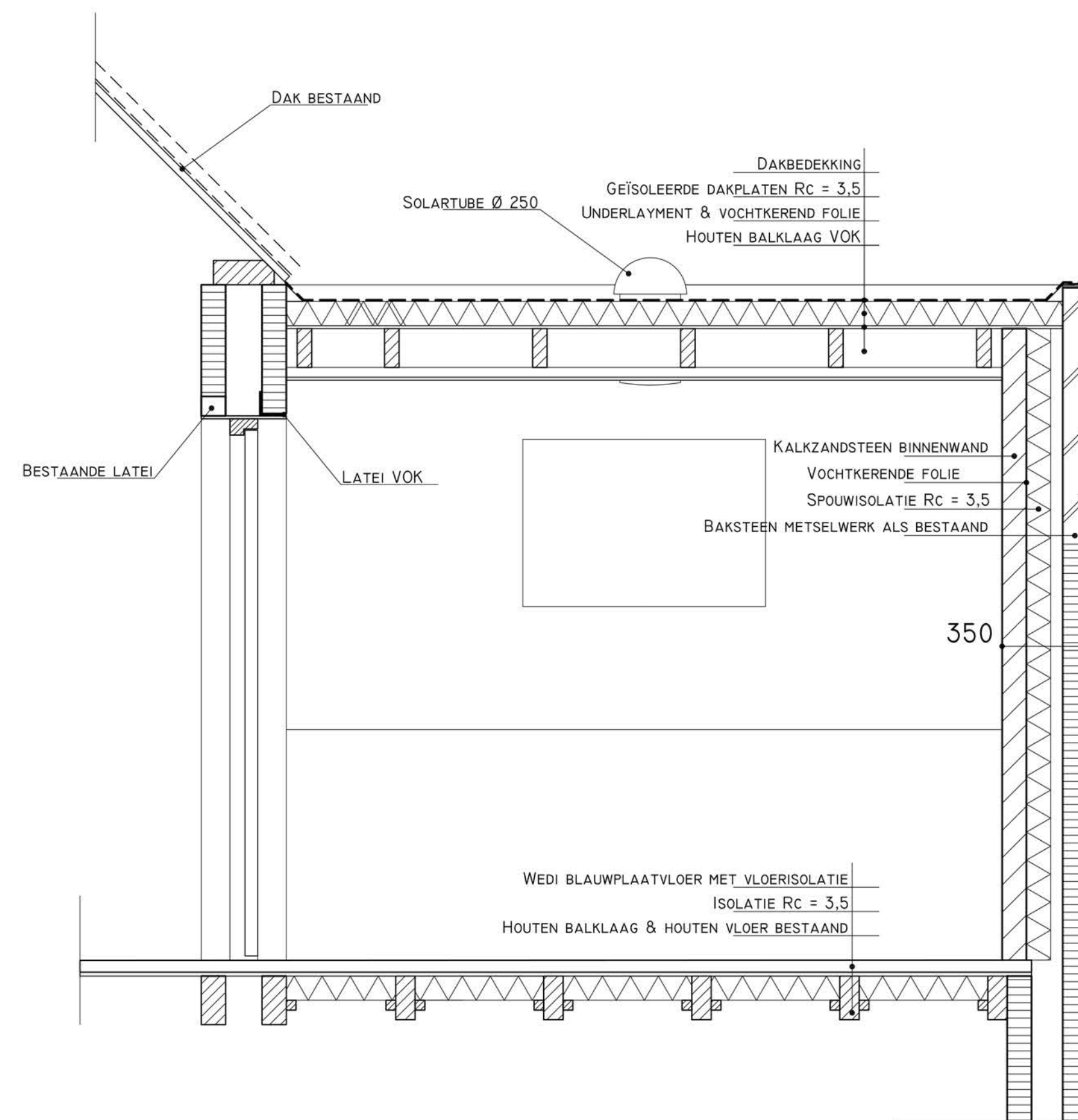
DOORSNEDE C-C' 1:20
