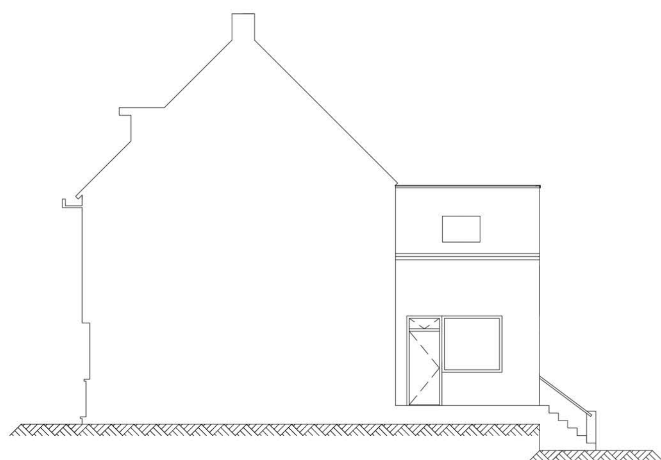
RECHTER ZIJAANZICHT
