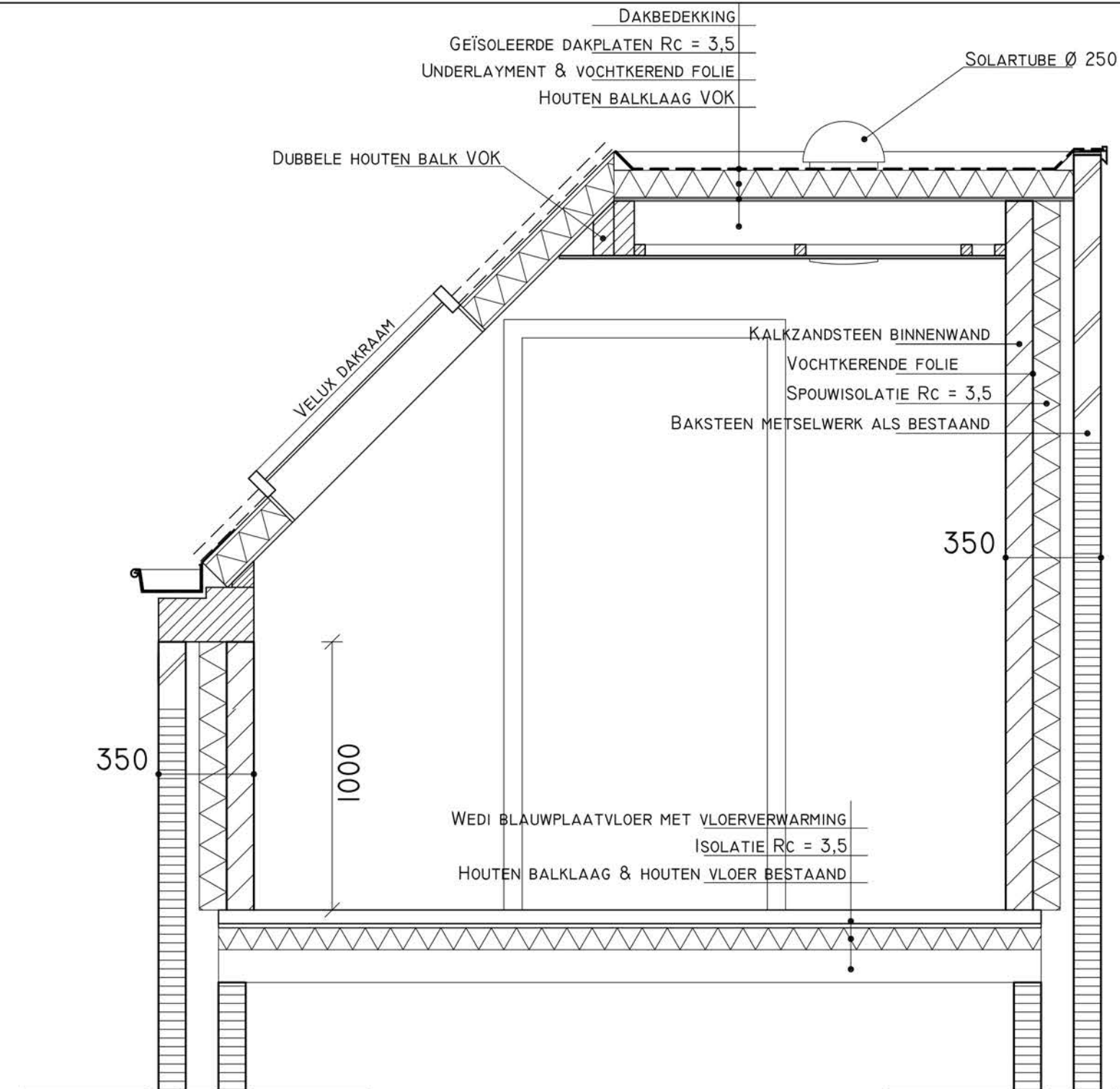
DOORSNEDE B-B'
