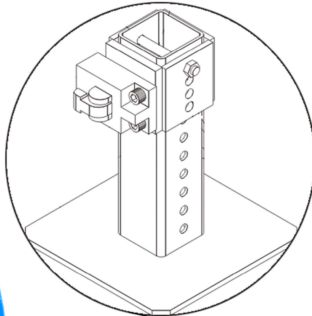
TANDEMLOC CONTAINER LEVELING LEG
